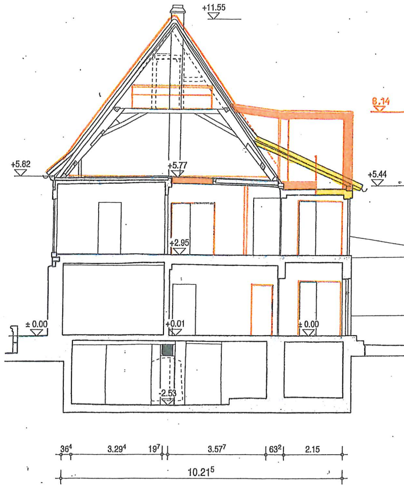
QUERSCHITT
